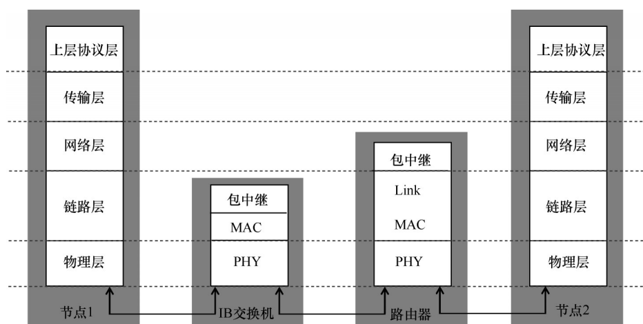
图5 IB协议栈
